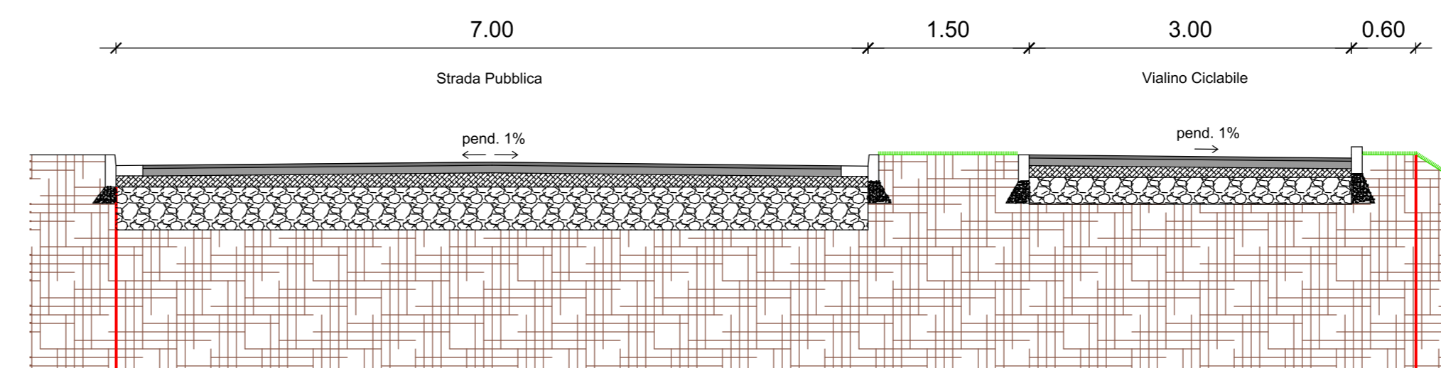
Particolare - Sezioni 2, 3, 4 Scala 1:50
