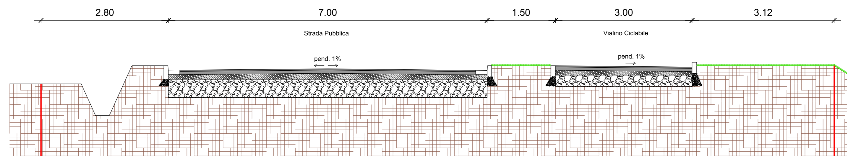
Particolare - Sezione 1 Scala 1:50
