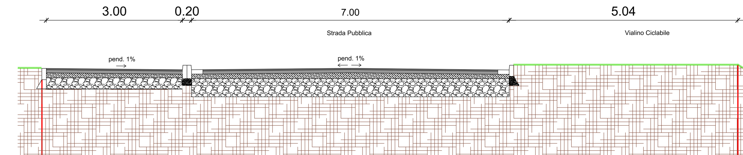
Particolare - Sezione 5 Scala 1:50
