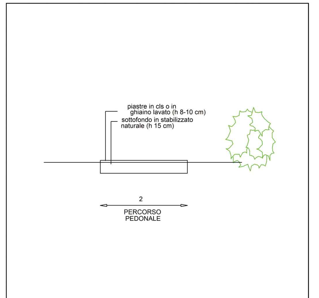
SEZIONE 2-2 PARTICOLARE B
