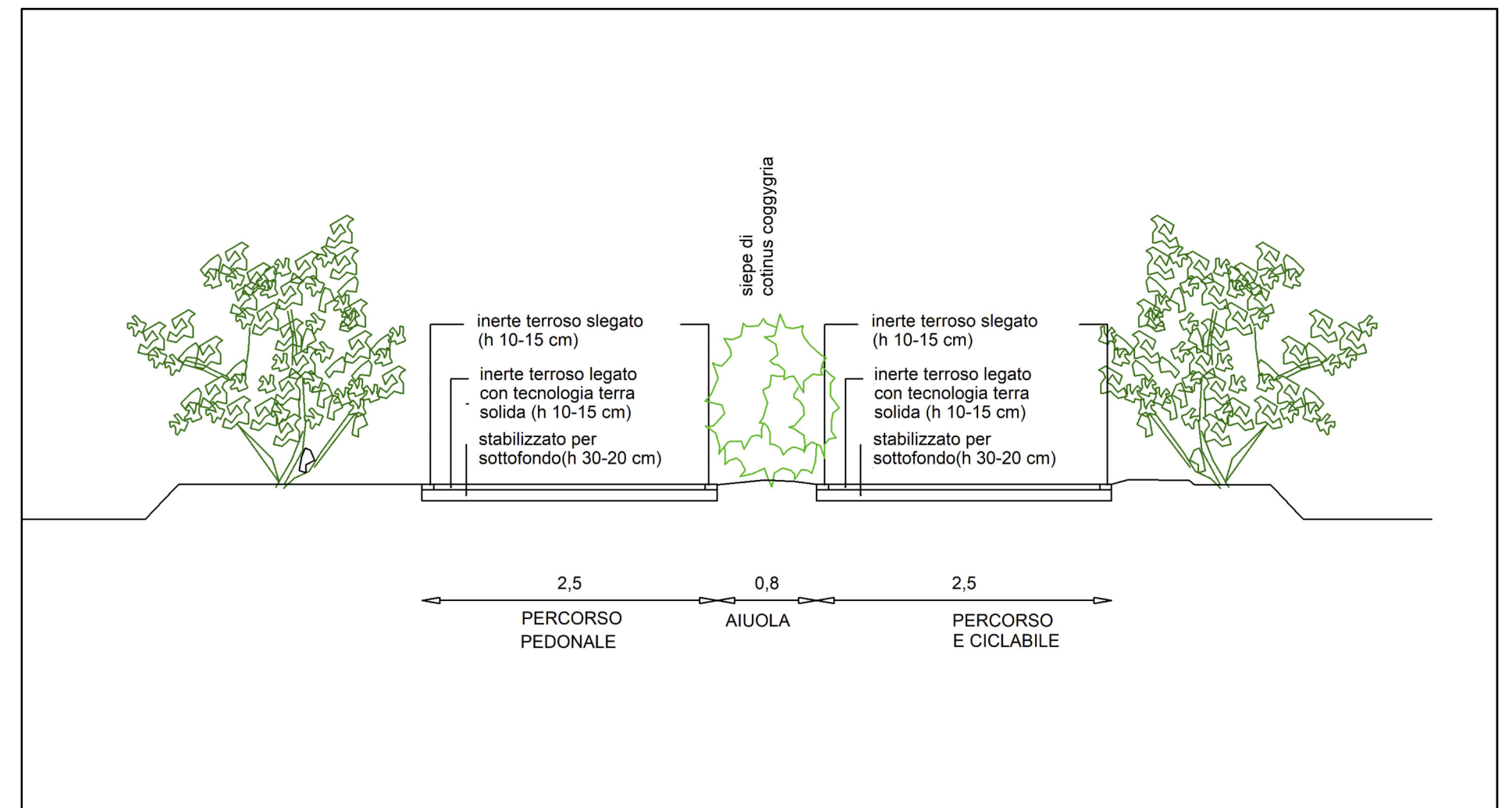
SEZIONE 1-1 PARTICOLARE A
